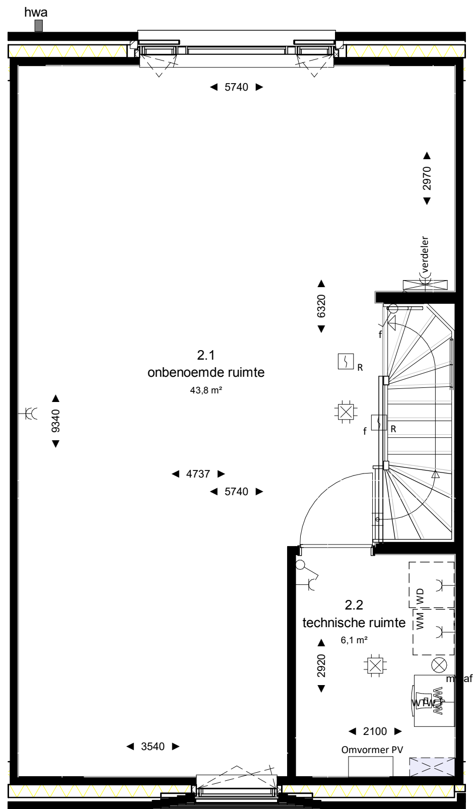
tweede verdieping
