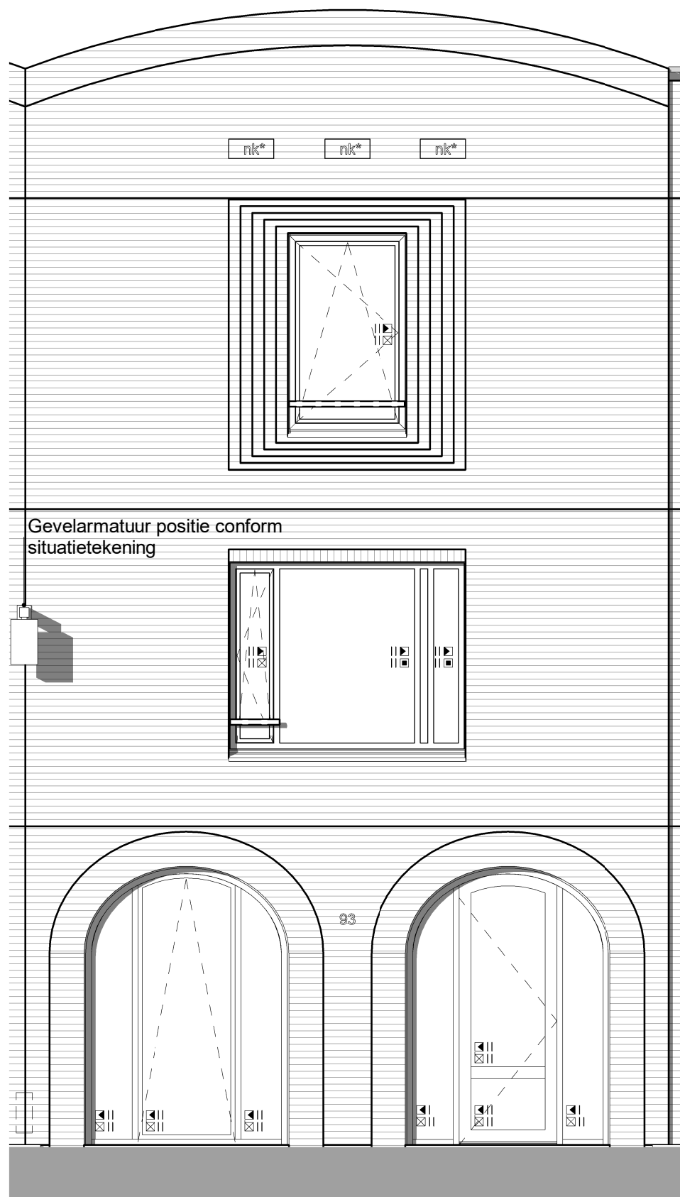
voorgevel
